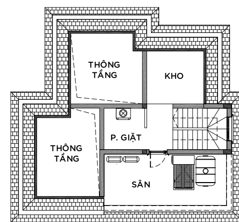
MẶT BẰNG TẦNG 4
