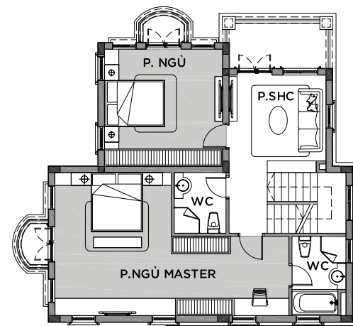
MẶT BẰNG TẦNG 3
