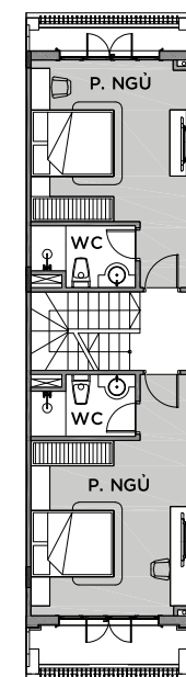
MẶT BẰNG TẦNG 2
