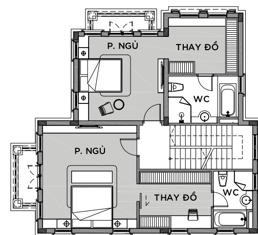
MẶT BẰNG TẦNG 2
